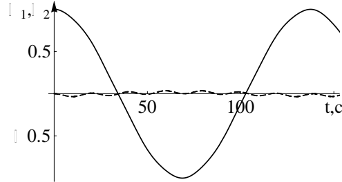
Рис. 1б. Зависимость \alpha_1 (штрих) и \alpha_2 (сплошная) от времени t , при kh = 1 для \zeta_1 = 0, \zeta_2 = 1, \rho_1 = 1, \rho_2 = 1.05
